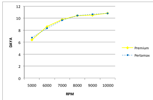
Gambar 4. Grafik Hasil Pengujian Daya
