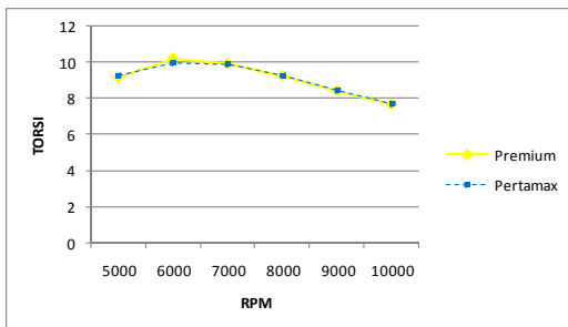
Gambar 3. Grafik Hasil Pengujian Torsi
