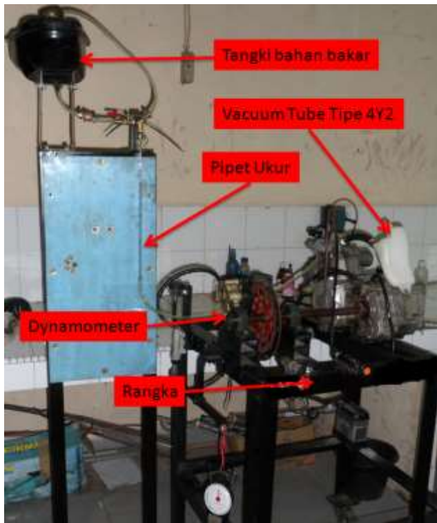
Gambar 2.1. Alat Uji Motor Bakar Bensin
