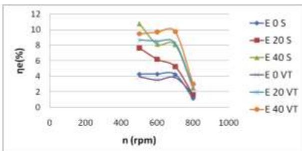
Gambar 3.4. Grafik ηe vs n
