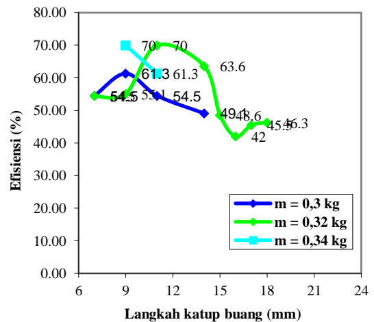
Gambar 8. Grafik hubungan antara efisiensi terhadap panjang langkah katup buang.
