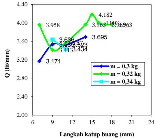
Gambar 7. Grafik hubungan antara laju aliran volume air yang dipompakan terhadap panjang langkah.
