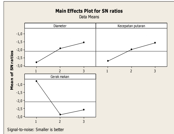
Gambar 1. Grafik S/N Rasio Kekasaran Permukaan
