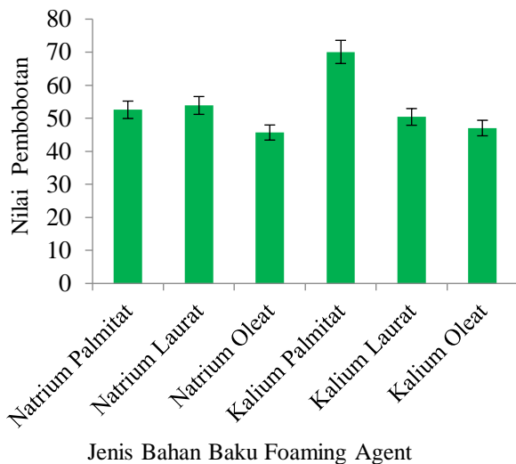
Gambar 2. Nilai pembobotan
