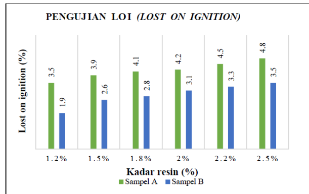
Gambar 5. Data hasil pengujian hasil pengujian LOI sampel A dan sampel B.
