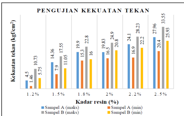
Gambar 4. Data hasil pengujian kekuatan tekan sampel A dan sampel B
