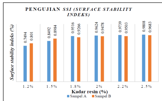
Gambar 6. Data hasil pengujian hasil pengujian SSI sampel A dan sampel B.
