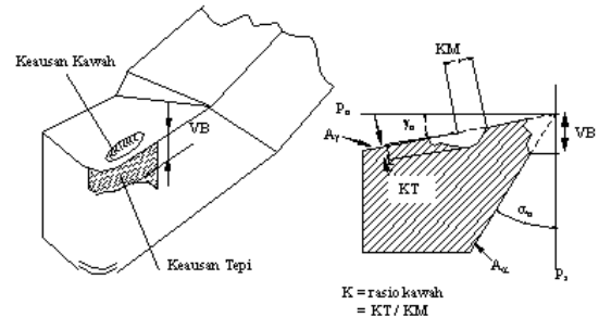
Gambar 1. Keausan Kawah dan Tepi [2]
