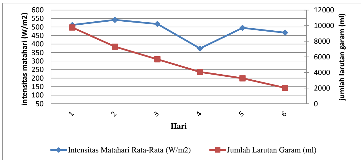
Gambar 4. Hubungan antara intensitas matahari dengan jumlah larutan garam
