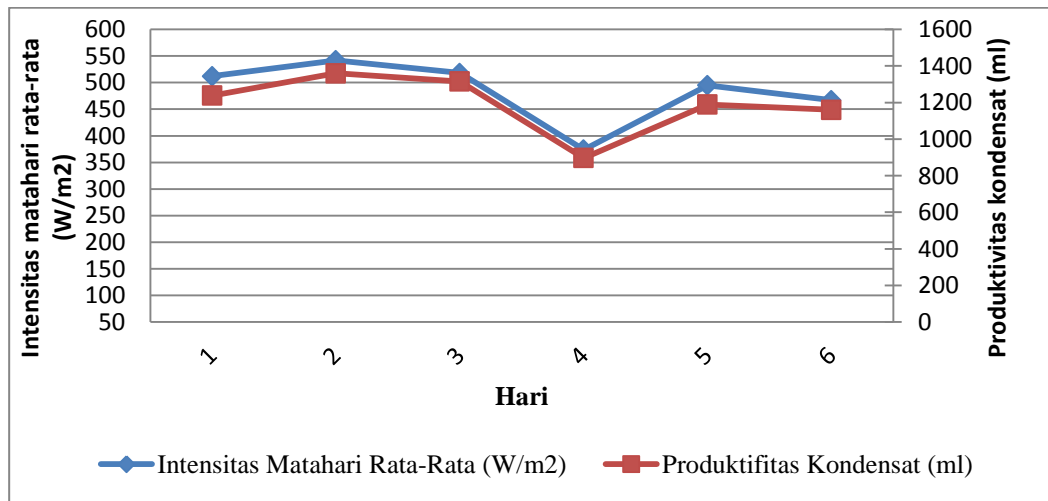
Gambar 3. Hubungan antara intensitas matahari dengan produktivitas kondensat
