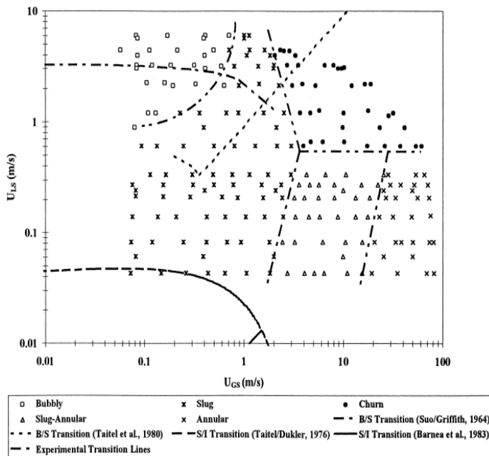
Gambar 4. Peta pola aliran dari Triplett dkk.[3] untuk aliran searah dalam pipa berdiameter dalam 1,097 mm.
