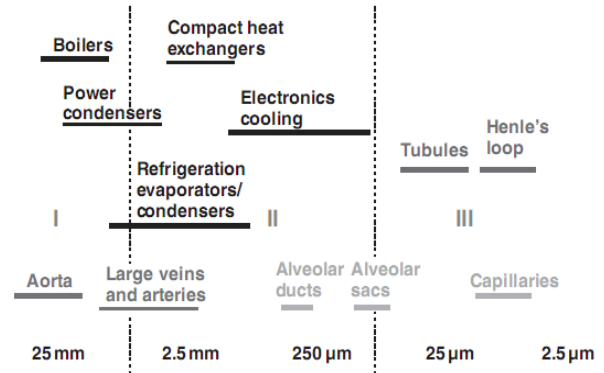
Gambar 2. Skema aplikasi aliran dua-fase berdasarkan ukuran saluran [5].
