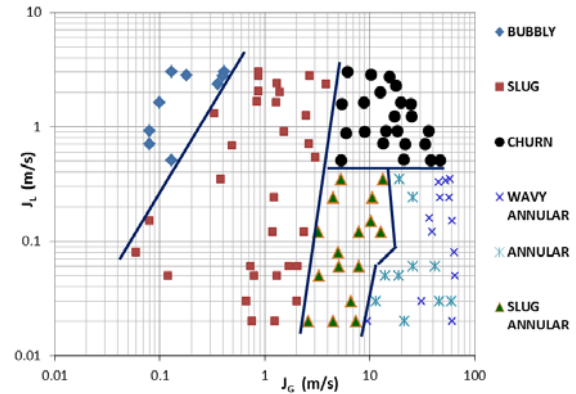
Gambar 8. Peta pola aliran dan garis transisi penelitian ini
