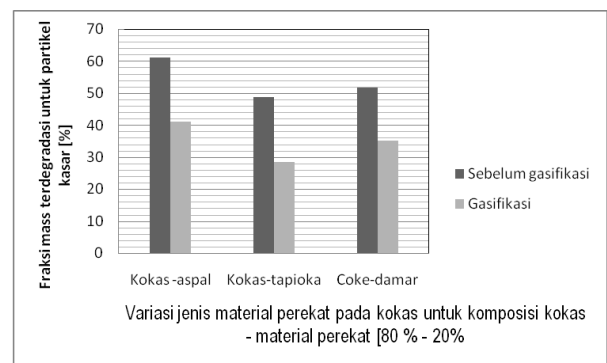
Gambar 5. Profil fraksi massa partikel besar dari briket kokas dengan jenis material perekat yang berbeda
