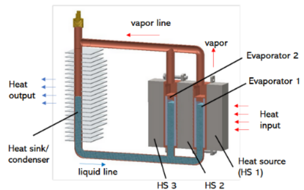
Gambar 1. Gambar 3D detail dari DE-LHP
